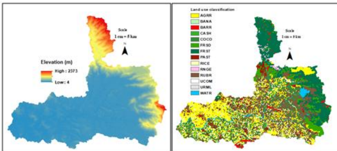
Fig. 2. DEM of the study area
